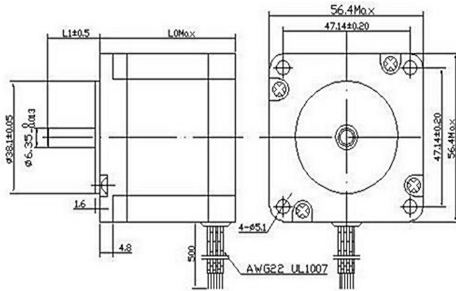
外形图 (FIGURE)
