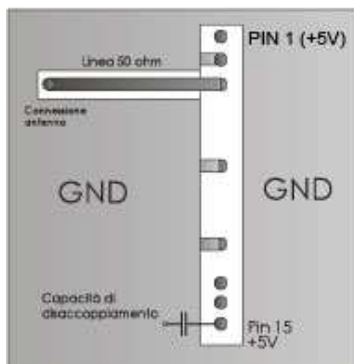
Fig. 2 - Lay-out consigliato per un corretto funzionamento del dispositivo
