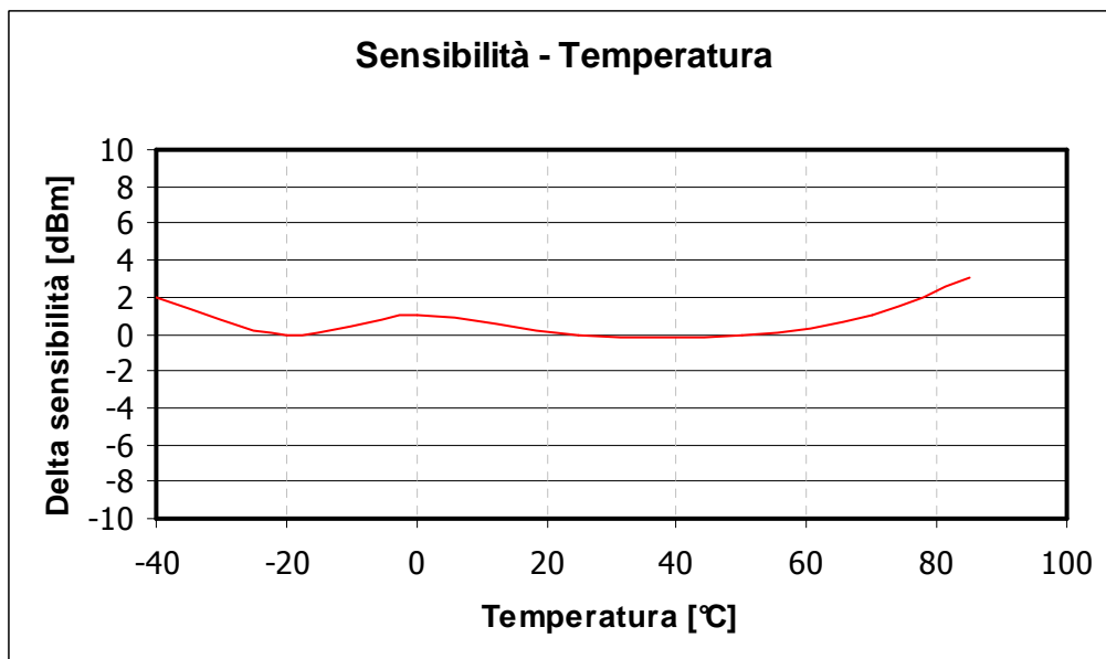
Fig. 4 – Delta sensibilità in funzione della temperatura
