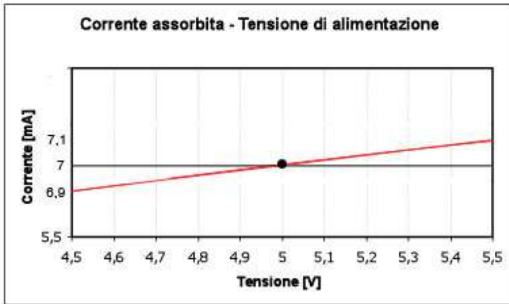
Fig. 3 – Andamento corrente in funzione della tensione
