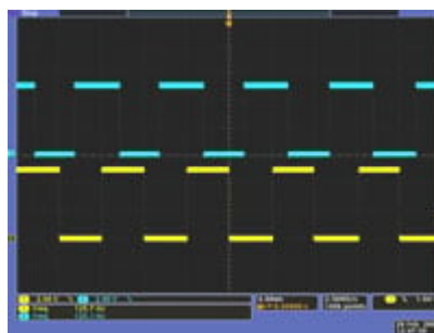
Immagine all'oscilloscopio delle uscite dell'encoder con la ruota che gira a 630 RPM
