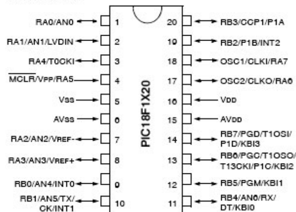
20-Pin SSOP
