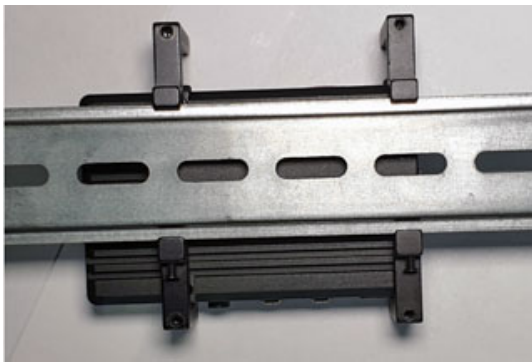
La Staffa montata su guida DIN
